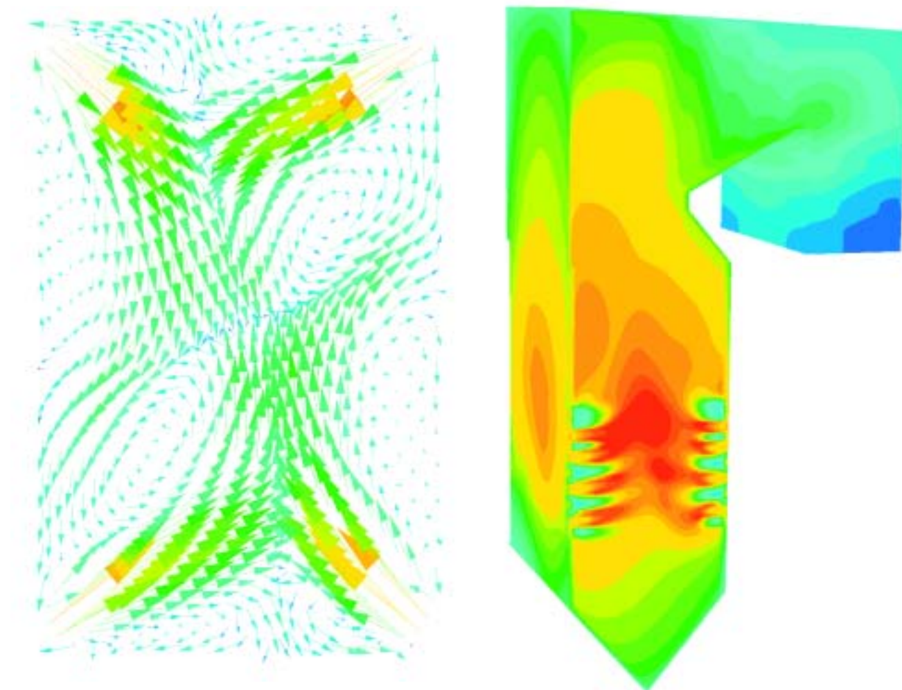
可変反応度木炭モデルを使用したフルスケールの T 型焚き産業用ボイラー(400MW)内の水平面上の温度分布と速度ベクトル
