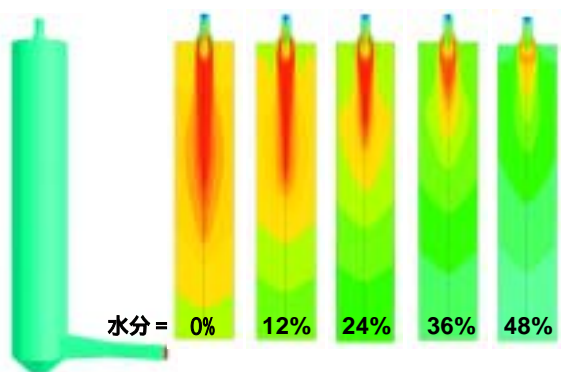
水分が NETL パイロットスケール燃焼器(110kW)内の温度に与える影響
