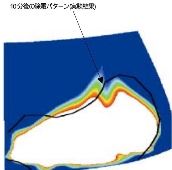
図2 CFDが予測した運転10分後の除霜パターンと実験データ(黒色の線)との比較
