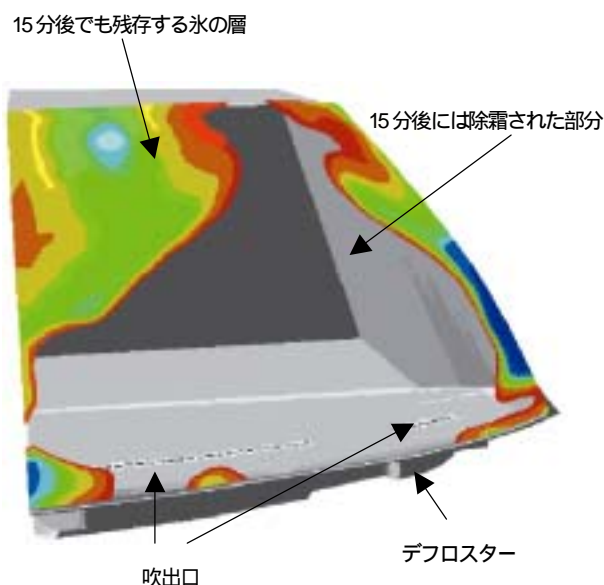
図1. 運転15分後のフロントガラス除霜パターンと車室内
